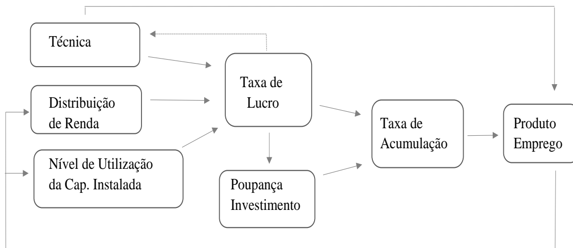
Diagrama 1: Relações de determinação em um modelo simples de crescimento
